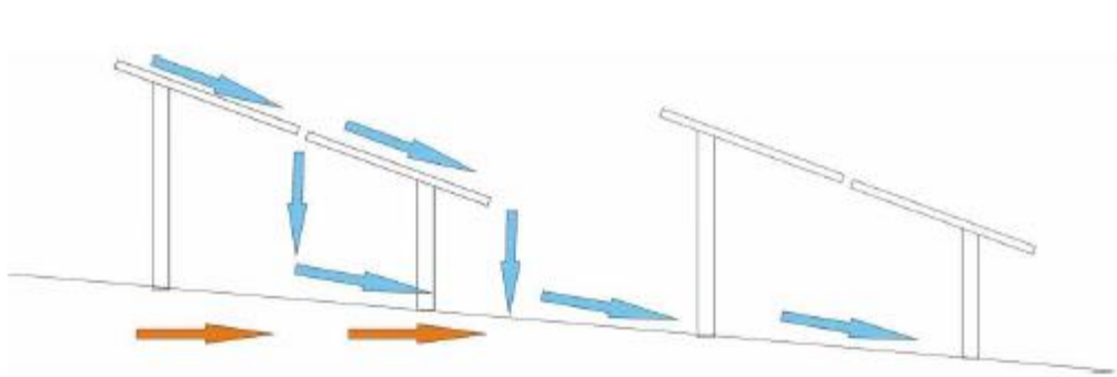
Abbildung 5: Lücken zwischen übereinander installierten PV-Modulen dienen als zusätzliche Tropfkanten
