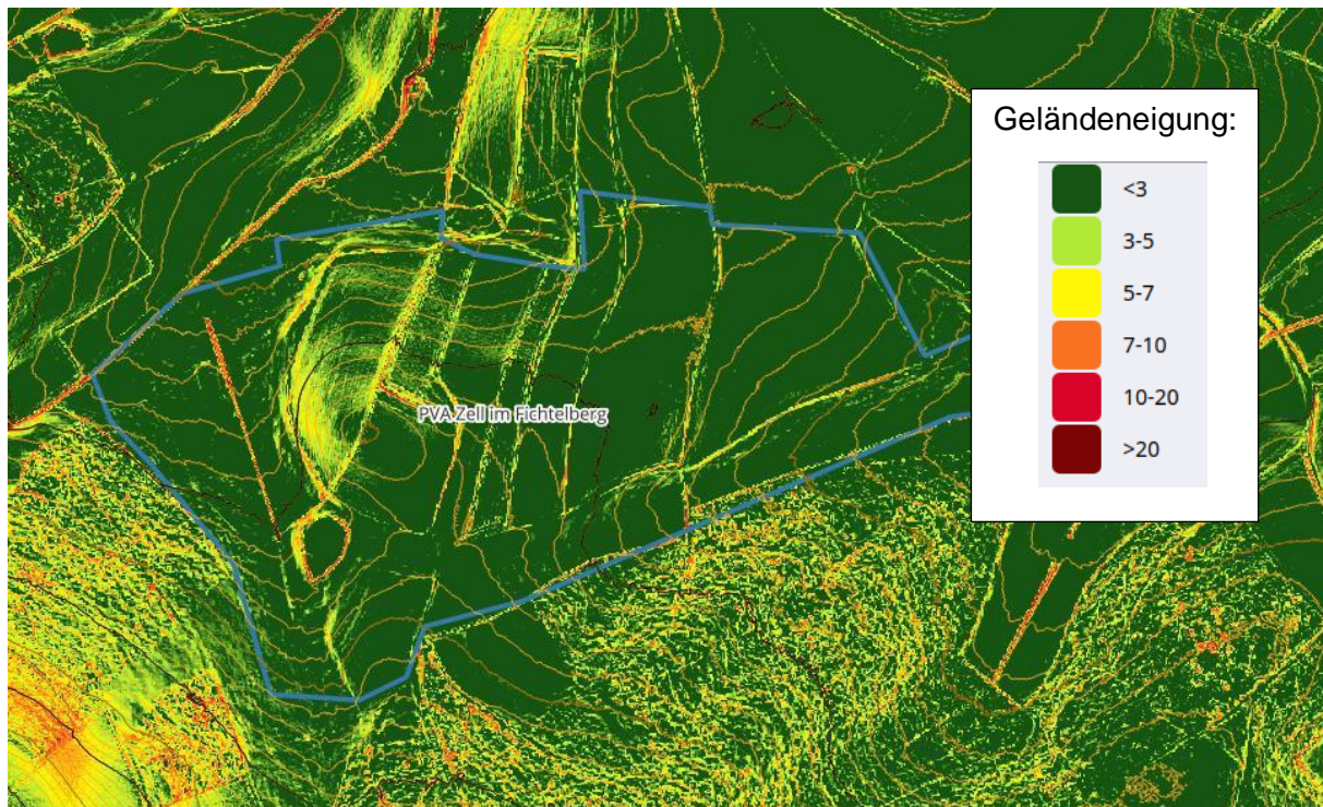
Abbildung 2: Hangneigung sowie Höhenlinien (schwarz: 10m, braun 5 m, gelb 1m) und Grenzen des Solarparks. Eigene Berechnungen basierend auf dem DGM1 Datenquelle: Landesamt für Digitalisierung, Breitband (Bayern)
