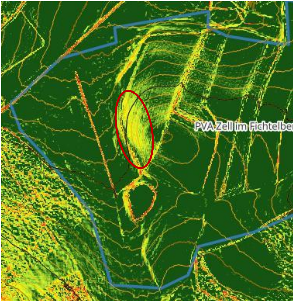
Abbildung 3: Kritischster Bereich der Anlage (rot umrandet), insbesondere, da hier die Tropfkanten der Module orthogonal zu den Höhenlinien stehen und somit Rinnenbildung möglich wäre. Allerdings sind die Neigungen selbst hier sehr moderat und somit nicht sehr kritisch
