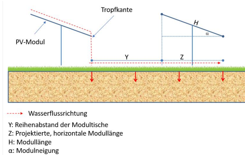
Abbildung 4: Schematische Darstellung des Regenwasserverlaufs an PV-Modulen auf Freiflächenanlagen – Quelle: Minnesota Pollution Control Agency (modifiziert)
